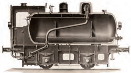
Schnittbild einer Dampfspeicherlok
