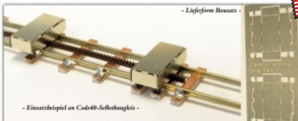
Nm-541.2: Montagelehre für Zahnstange Strub/von Roll, 2 Stück im Bausatz, für Code40-Gleise (Selbstbau, Kleinserie)
