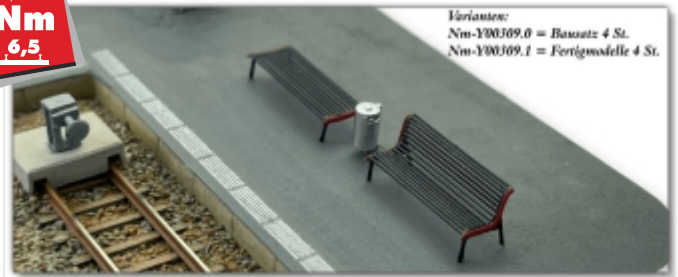
Nm-Y00309: moderne Sitzbänke, je 2 St. mit und ohne Rückenlehne, Ätzbausatz oder Fertigmodelle (bitte angeben)
