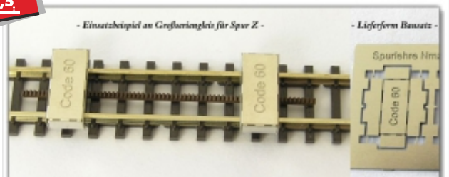
Nm-541.3: Montagelehre für Zahnstange Strub/von Roll, 2 Stück im Bausatz, für Code60-Gleise (z.B. Märklin, Peco)
