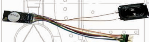
83450 LOKSOUND DECODER ALCO 1300 ESCALA HO - 8 PINS ALTAVOZ /SPEAKER Ø23mm
